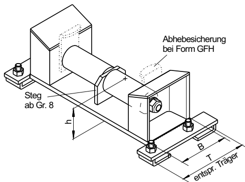
Typ 118-305P GFH, Gr. 5-11 Rollenlager mit seitlicher Führung und Abhebesicherung nur in Kombination mit Gleitunterstützung Typ 180 HS/ Katalogseite 120 sowie Typ 171-... HS/Katalogseite 159 + 160 verwendbar
