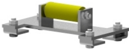
Typ 118-305P GOF, Gr. 2-11 Rollenlager ohne seitliche Führung
