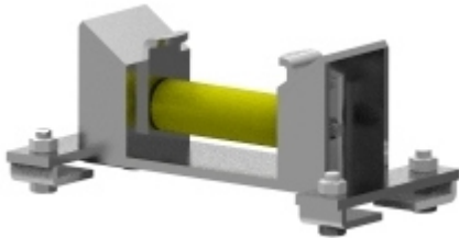
Typ 118-305P GFH, Gr. 5-11 Rollenlager mit seitlicher Führung und Abhebesicherung nur in Kombination mit Gleitunterstützung Typ 180 HS/ Katalogseite 120 sowie Typ 171-... HS/Katalogseite 159 + 160 verwendbar
