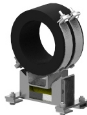
Rollenlager Typ 118-305P GF in Kombination mit Kältegleitunterstützung Typ 171-2 / s.S. 160
